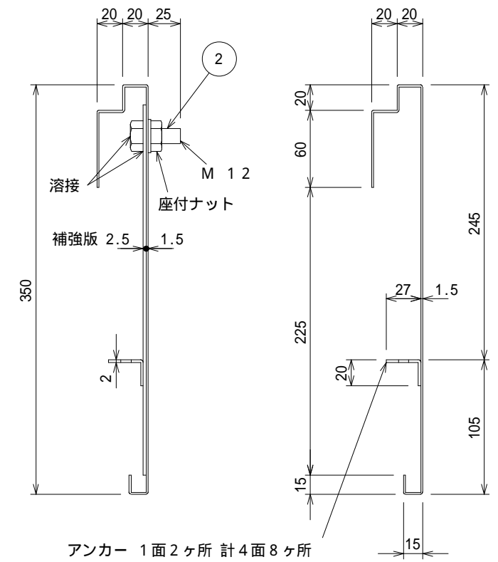
本体断面図 S = 1/4
